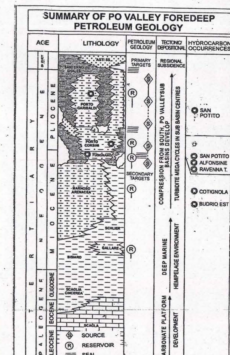
FIG.6 STRATIGRAFIA
