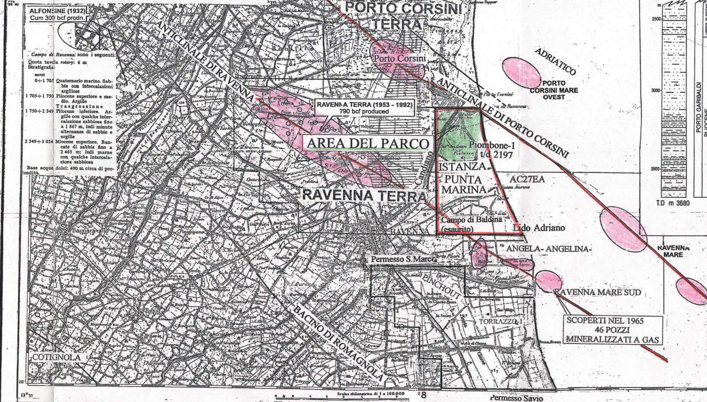
FIG.1 CARTA GEOLOGICA E MINERARIA
