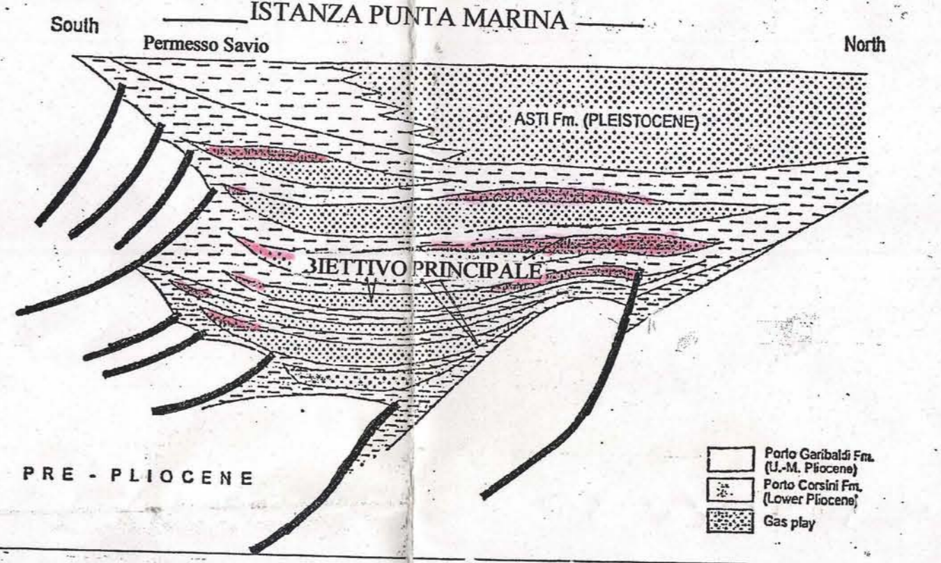
FIG.8 SEZIONE SCHEMATIZATA ATTRAVERSO L'ISTANZA PUNTA MARINA
