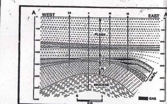
FIG.5 CAMPO DI RAVENNA TERRA
