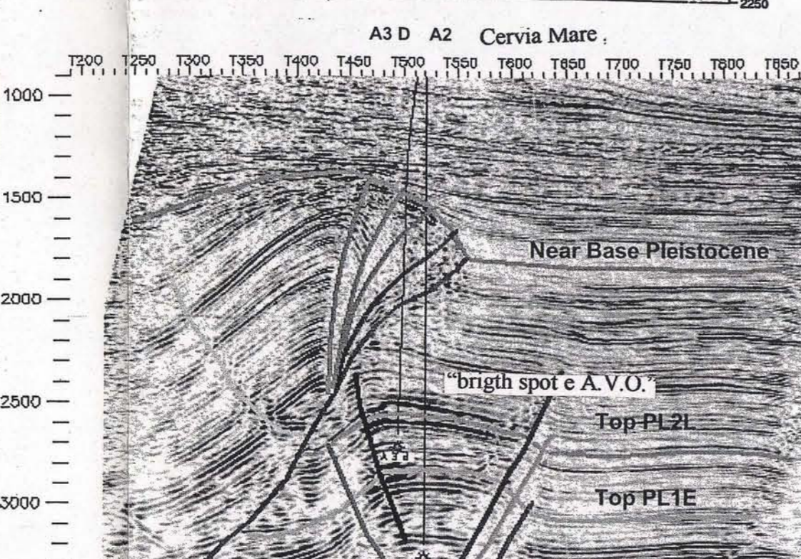
FIG.10 ESEMPIO DI SEZIONE GEOLOGICA E GEOFISICA NEI CAMPI DELLA ZONA
