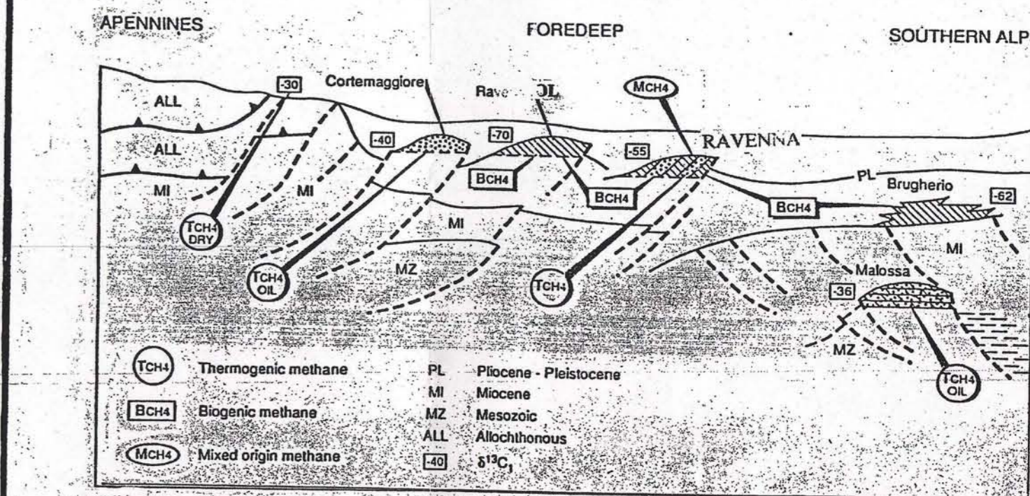
FIG.4 SCHEMA STRUTTURALE DELLA PIANURA PADANA ORIENTALE
