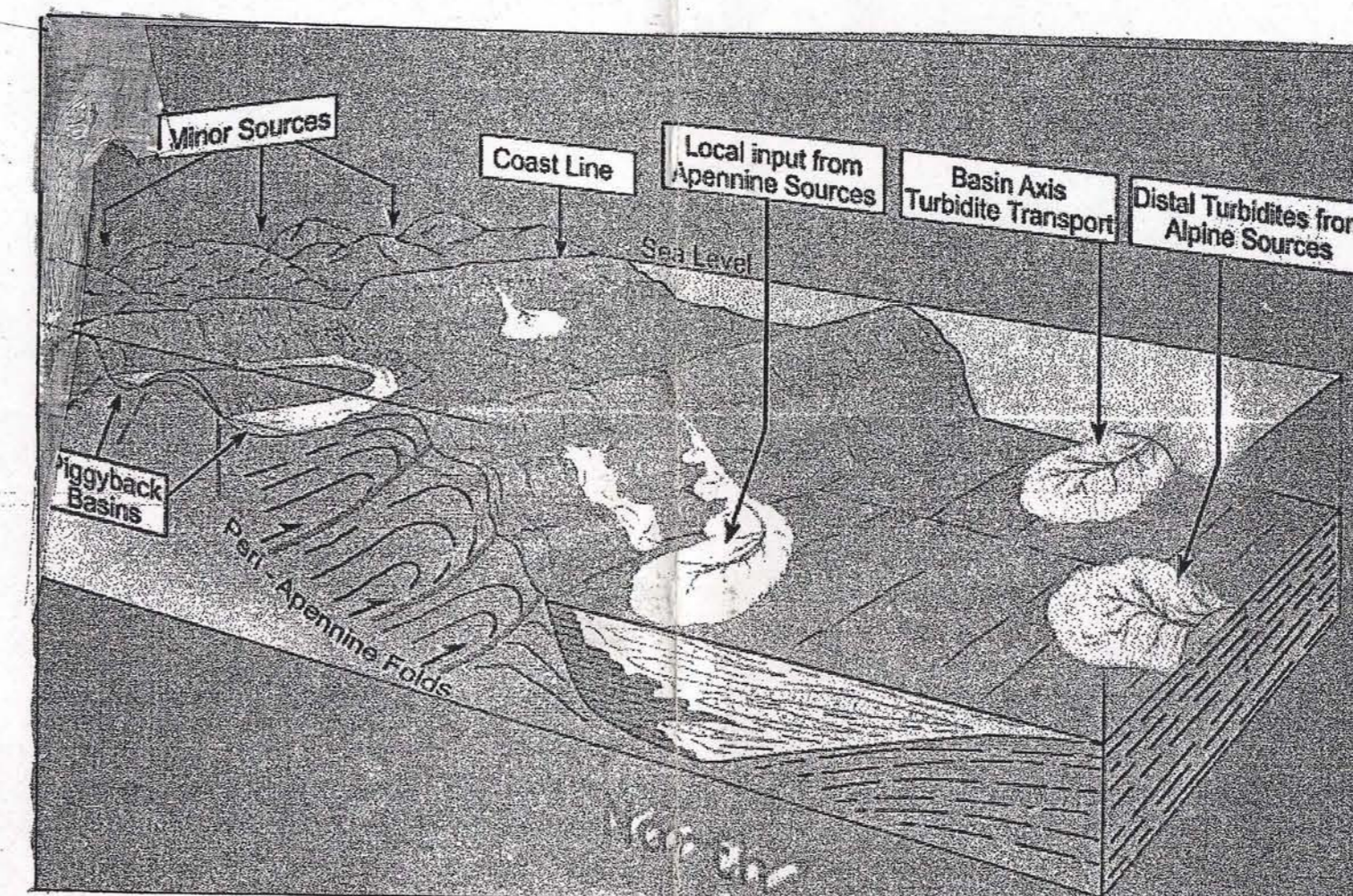
FIG.8 SEZIONE SCHEMATIZATA ATTRAVERSO L'ISTANZA PUNTA MARINA
