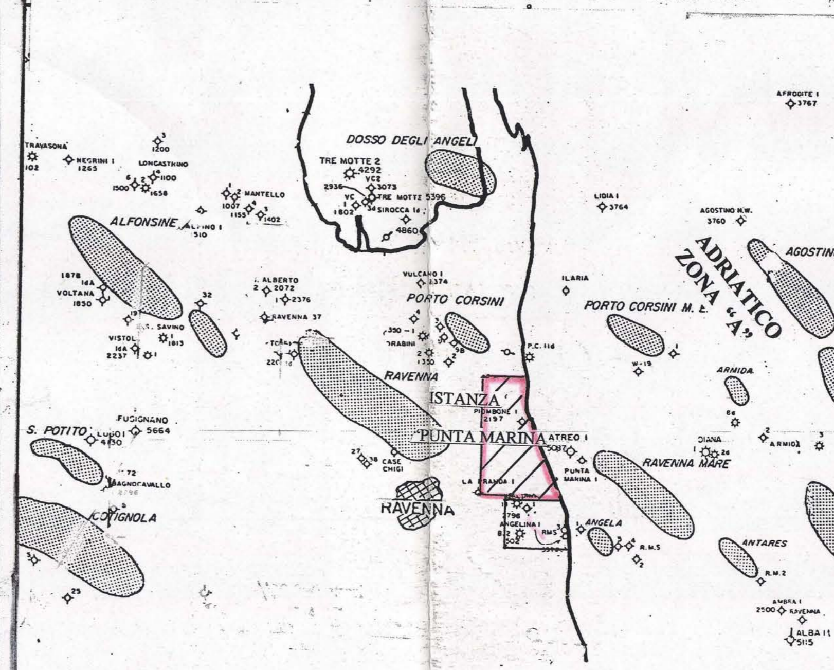
FIG.7 SOMMARIO DEI CAMPI DELLA PADDANA EST
