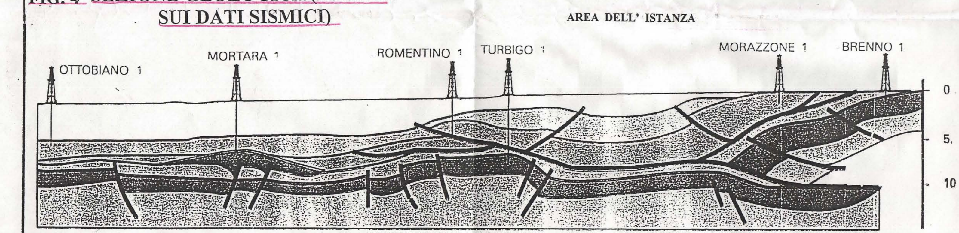
FIG. 5 STRATIGRAFIA DEL BACINO LOMBARDO
