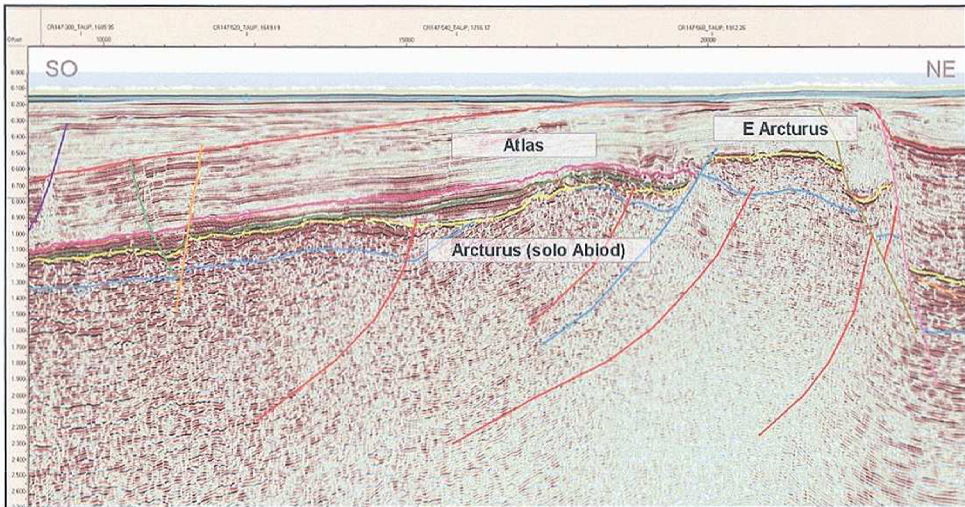
Figura 11 - Linea sismica CR147-180
