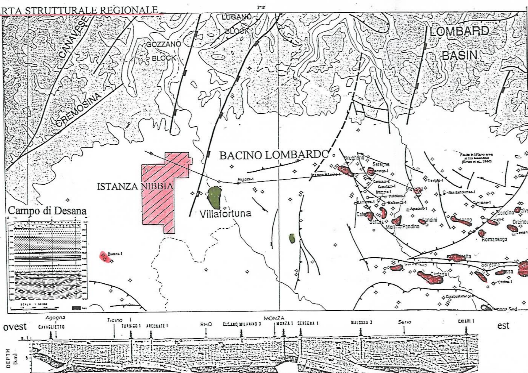
FIG. 10 CARTA STRUTTURALE REGIONALE
