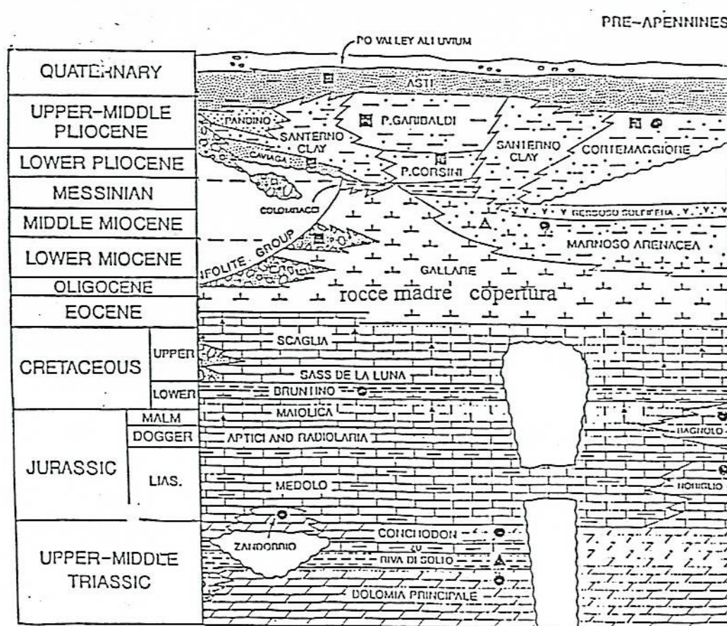
FIG. 11 STRATIGRAFIA DELLA PADANA OCCIDENTALE
