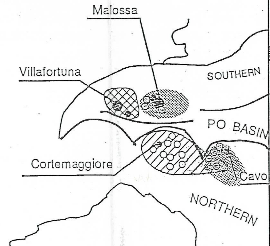
Fig. 7 ROCCIA MADRE "SOURCE KITCHENS"-PADANA OCCIDENTALE
