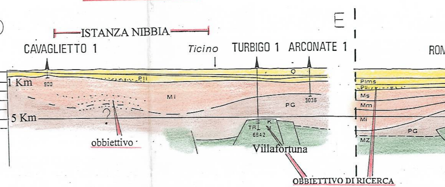
Fig. 7 ROCCIA MADRE "SOURCE KITCHENS"-PADANA OCCIDENTALE
