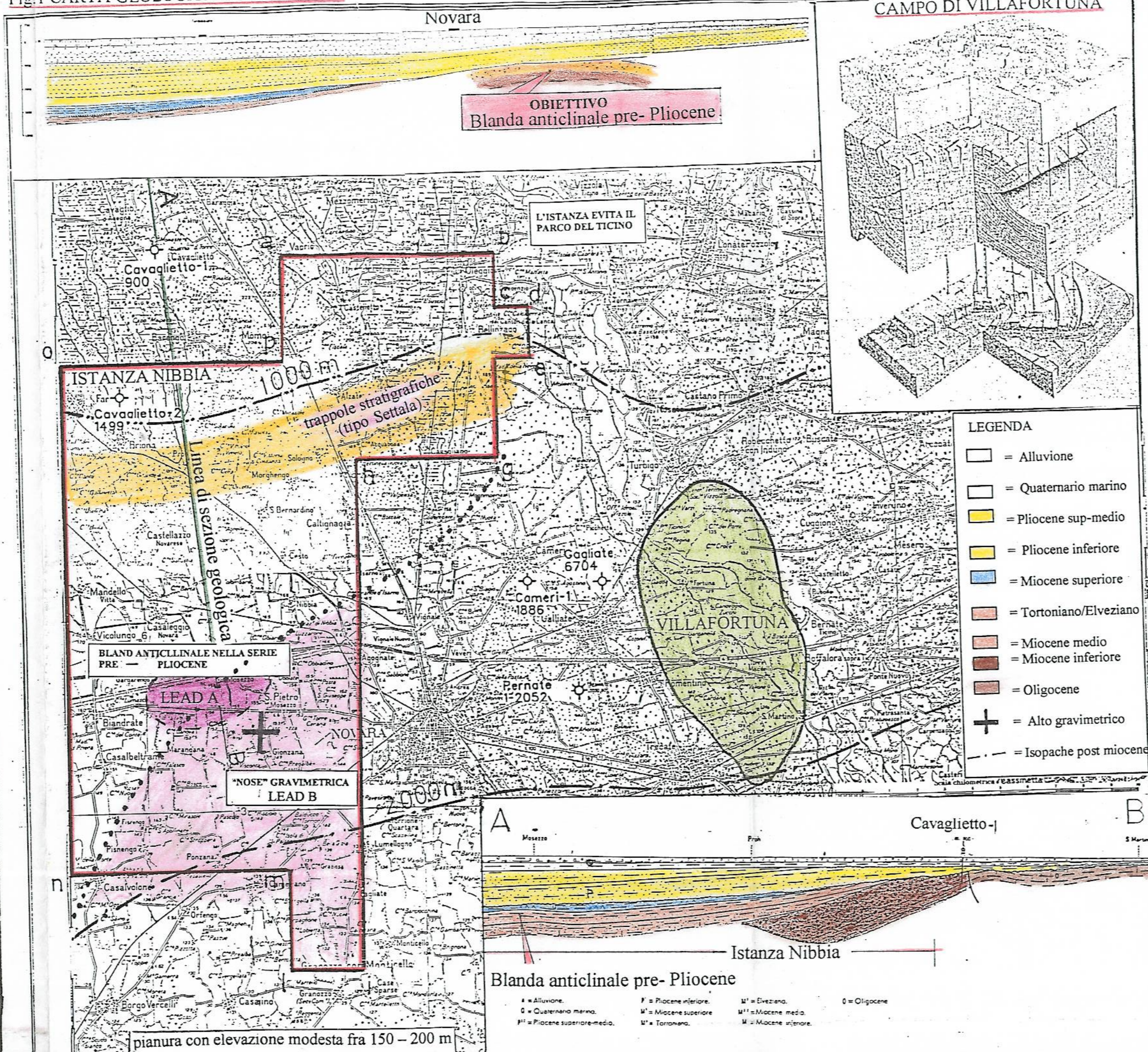
Fig. 1 CARTA GEOLOGICA E MINERARIA
