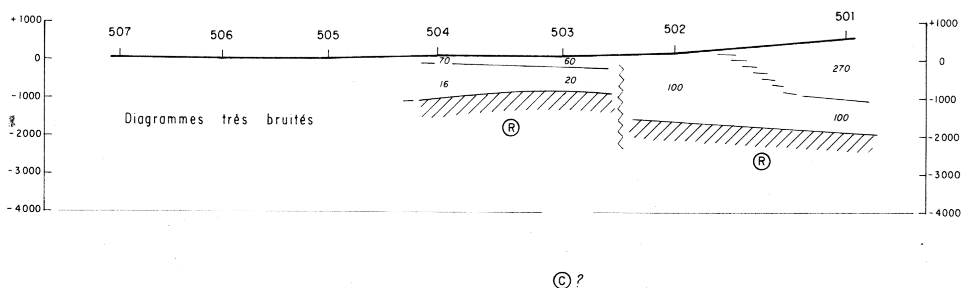
Profil 500
