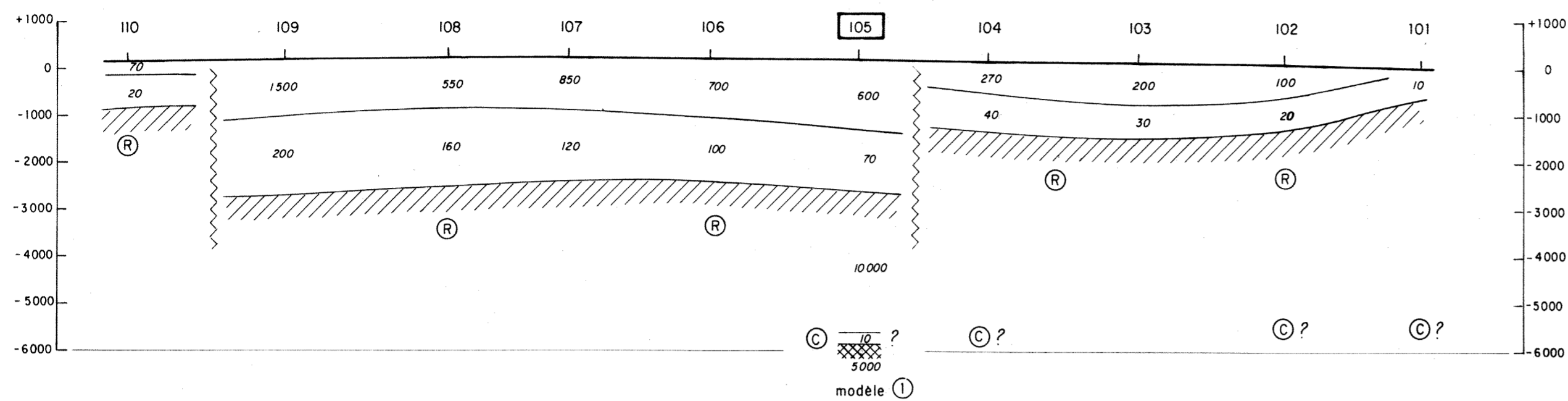
Profil 200
