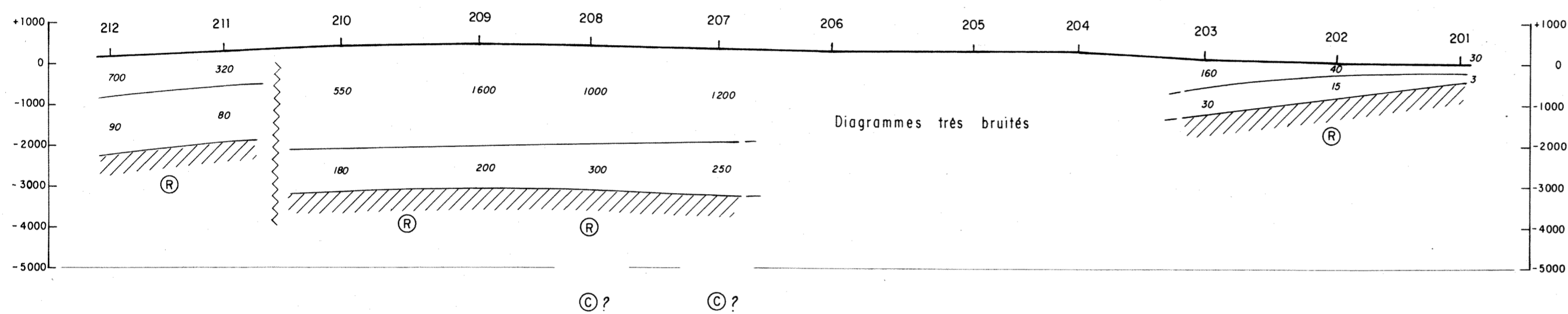
Profil 200
