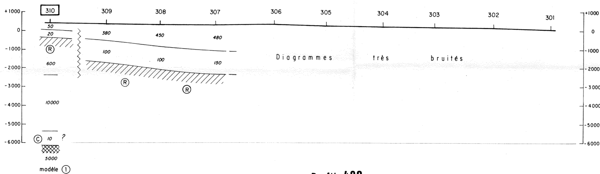
Profil 400
