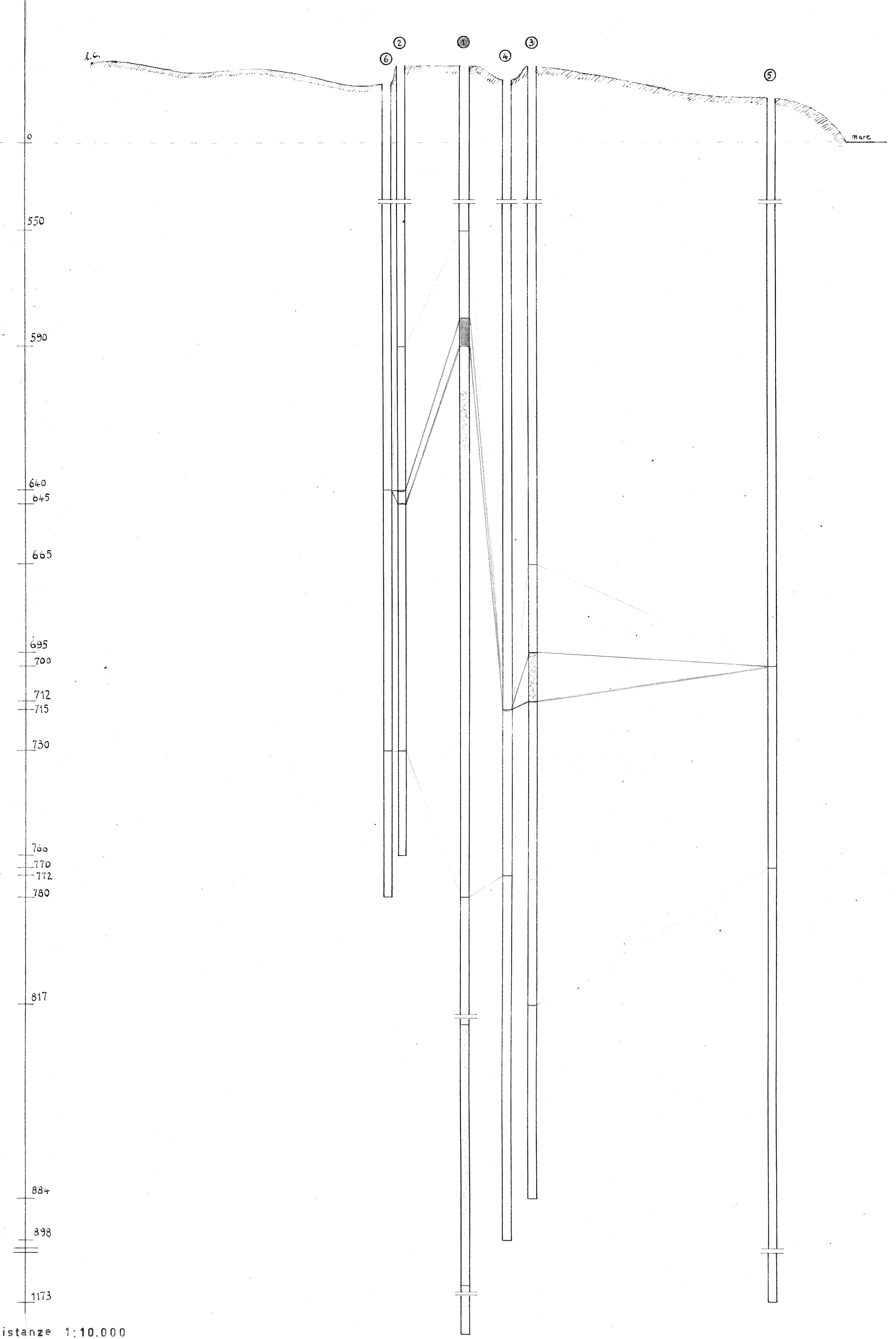
sezione C-D parallela al piano di faglia
