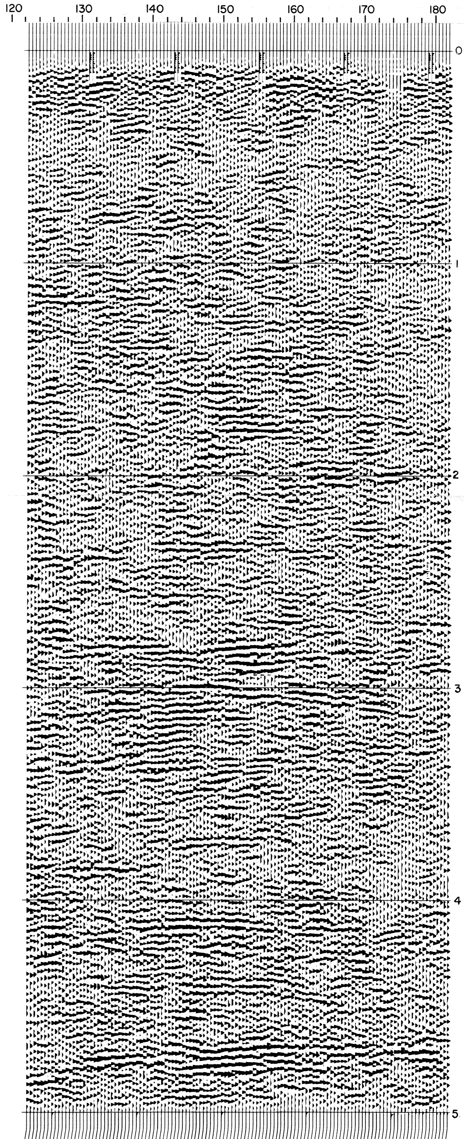
STACK-T.V.FILTER-T.V.EQUALISATION-COHERENCY SCALING
