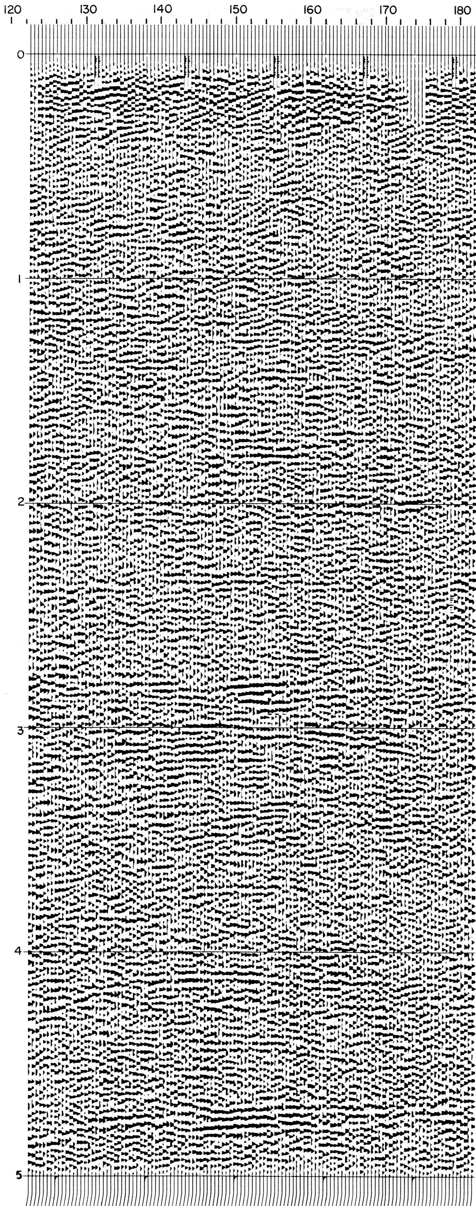
STACK-T.V.FILTER-T.V.EQUALISATION
