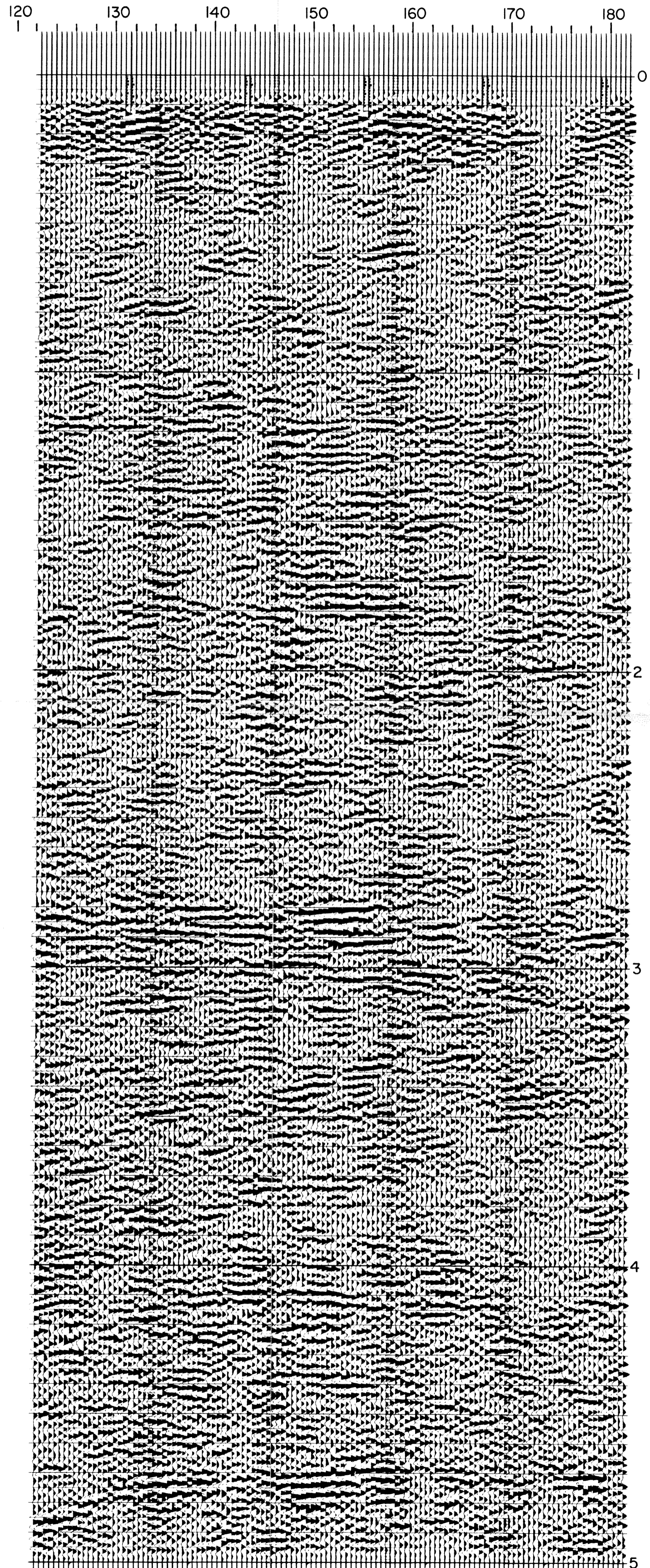
STACK-T.V.FILTER-T.V.EQUALISATION-COHERENCY SCALING
