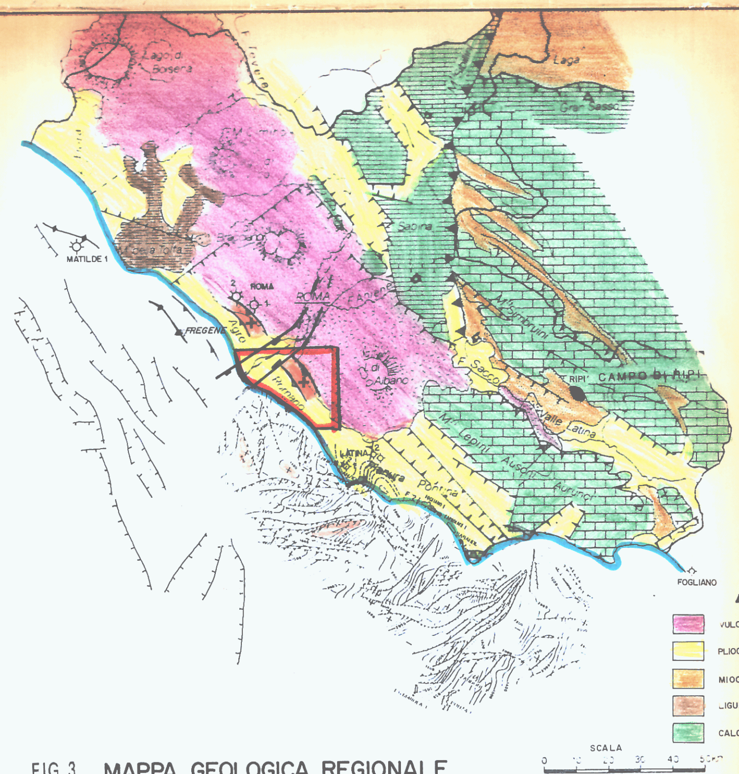
FIG. 3 MAPPA GEOLOGICA REGIONALE
